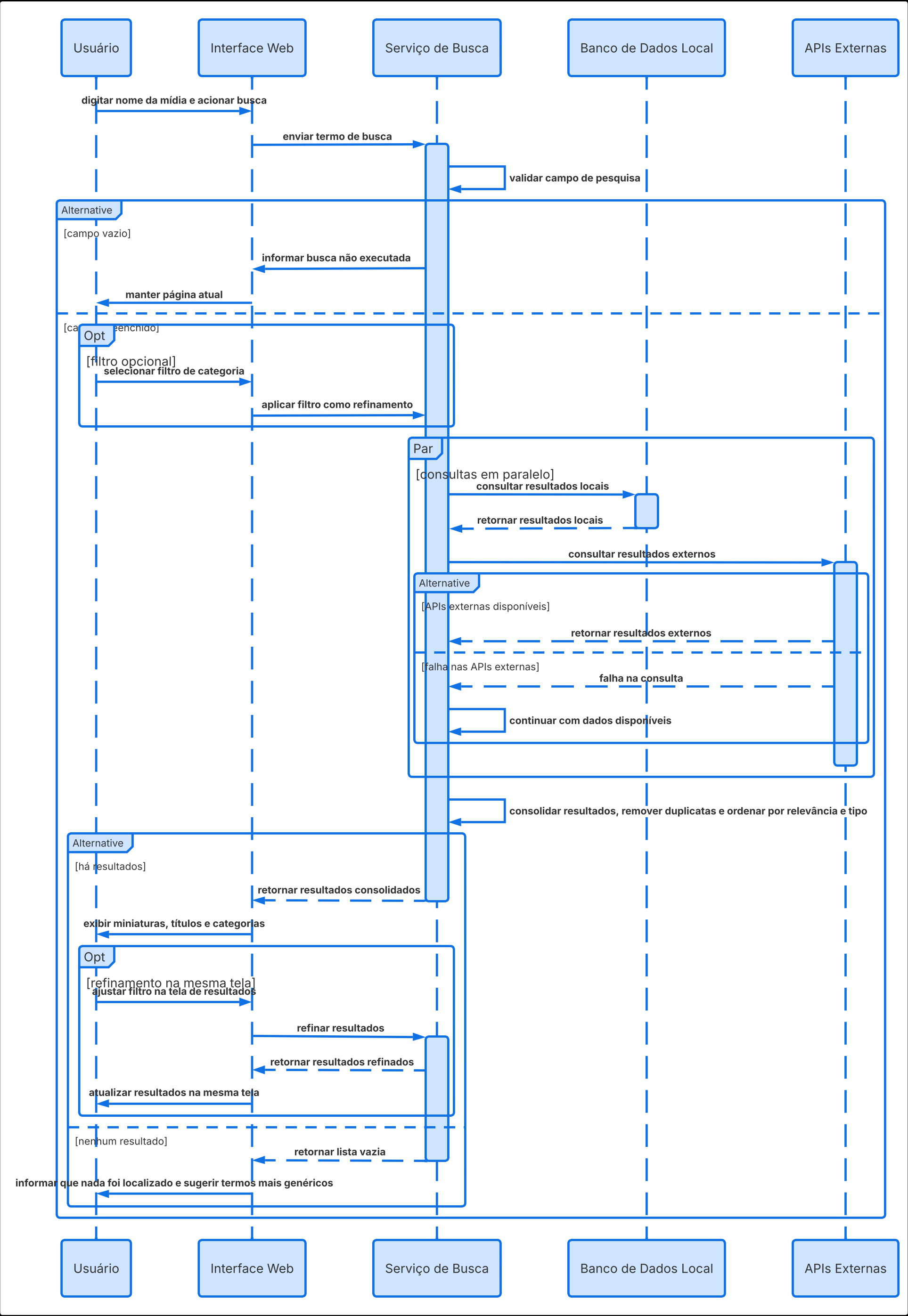
Diagrama de Sequência - Busca de Mídia
